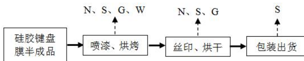
图 3-3 项目硅胶键盘膜生产工艺及产污环节流程图
