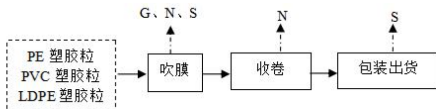
图 3-3 项目包装膜生产工艺及产污环节流程图
