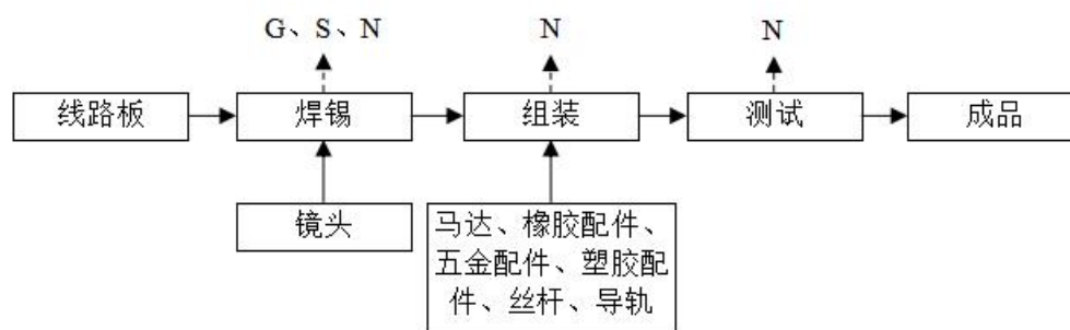
图 3-2 项目生产工艺流程及产污环节图
