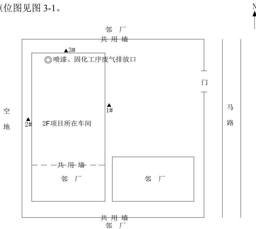
图 3-1 厂区平面布置及监测点位
