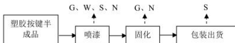
图 3-2 按键生产工艺及产污环节图
